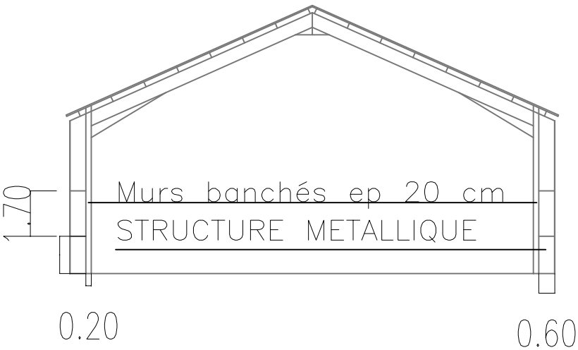
COUPE HANGAR N° 8
